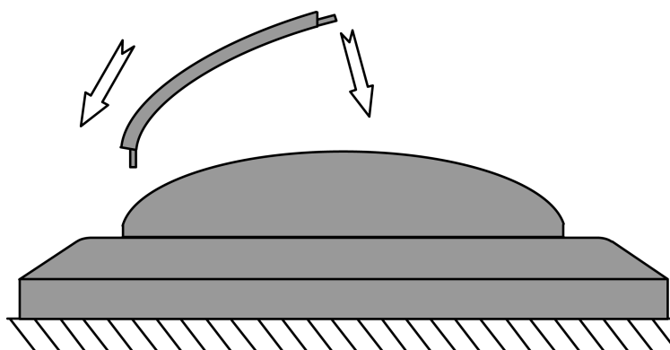
Bild 12: Abdeckblende 90° montieren
