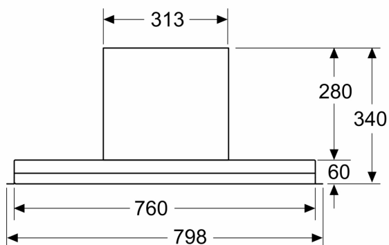
Maße in mm Frontansicht
