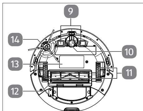
Fig. 3 – Parte inferior
