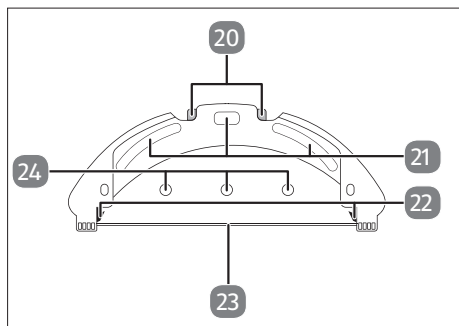
Afb. 6 – Dweilopzetstuk
