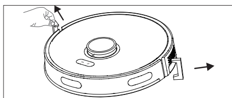
Fig. 9 – Rimozione della protezione per il trasporto
