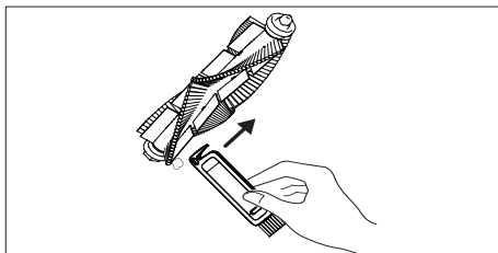
Abb. 34 – Bürste reinigen
