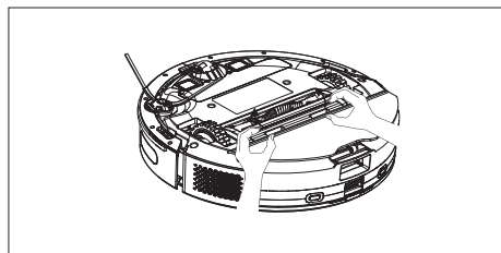
Abb. 33 – Bürste entfernen
