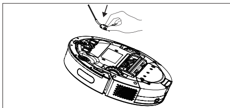
Afb. 10 – Zijborstel plaatsen
