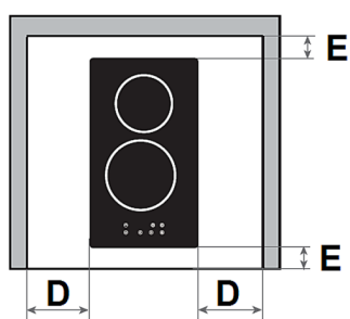
ERFORDERLICHER MINDESTFREIRAUM UM DIE EINBAUÖFFNUNG HERUM:
