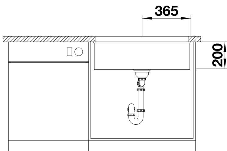
Frontansicht
