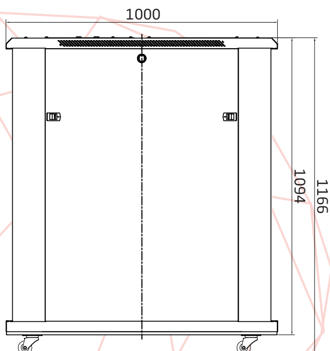
Seitenansicht
