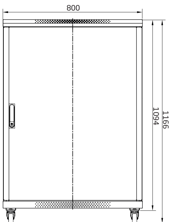
Hinteransicht
