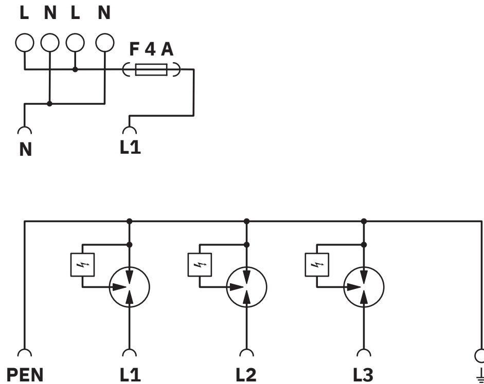
Schaltplan
