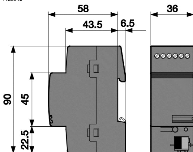
Maßbild
