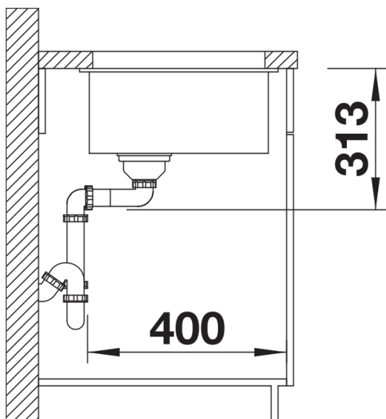
Seitenansicht
