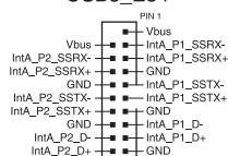
USB3_E34
