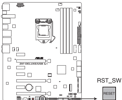
Z97-DELUXE/USB 3.1 Reset button
