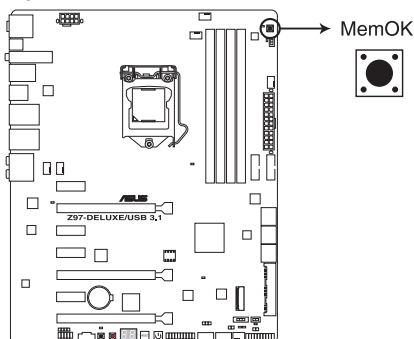
Z97-DELUXE/USB 3.1 MemOK! button
