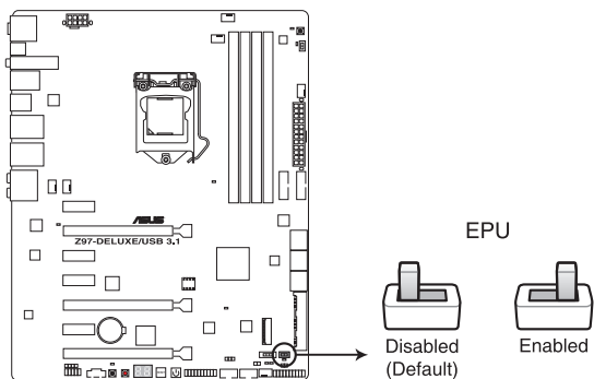
Z97-DELUXE/USB 3.1 EPU switch
