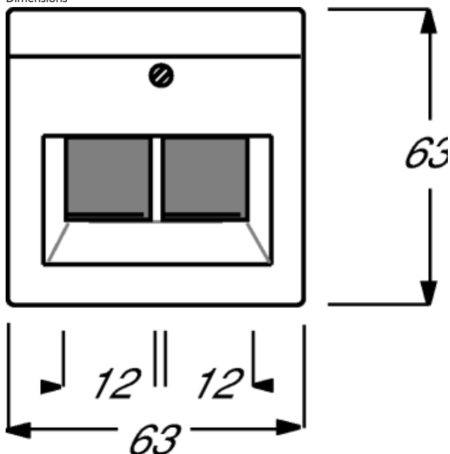
Dimensions
