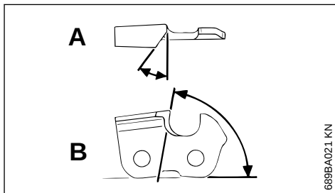
A Schärfwinkel
