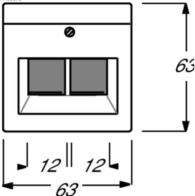
Maßbild
