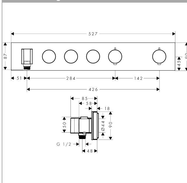
Maßzeichnung
