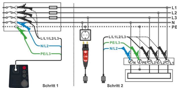
Abbildung 7.73: AUTO TT-Messung
