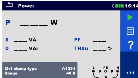
Abbildung 7.53: Menü Leistung
