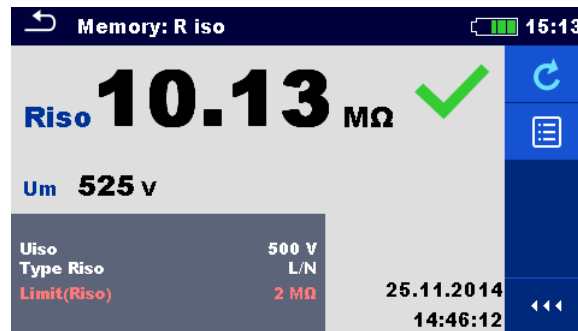
Abbildung 6.12: Speicherbildschirm einer Messung, Beispiel für Isolationswiderstandsmessung
