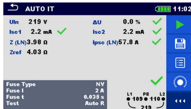
Abbildung 7.83: Beispiel für ein Ergebnis der AUTO IT-Messung
