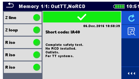
Abbildung 8.9: Speicherbildschirm der Auto Sequence®
