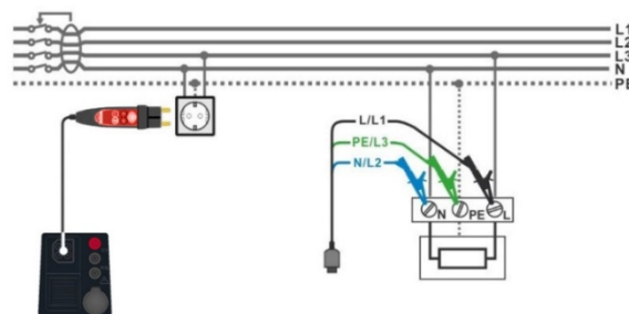
Abbildung 7.34: Anschluss des Commander-Prüfsteckers und der 3-Leiter-Prüfleitung
