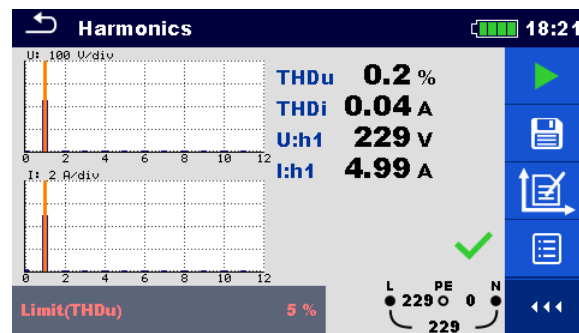
Abbildung 6.5: Beispiel für ein Ergebnis der Oberwellenmessung
