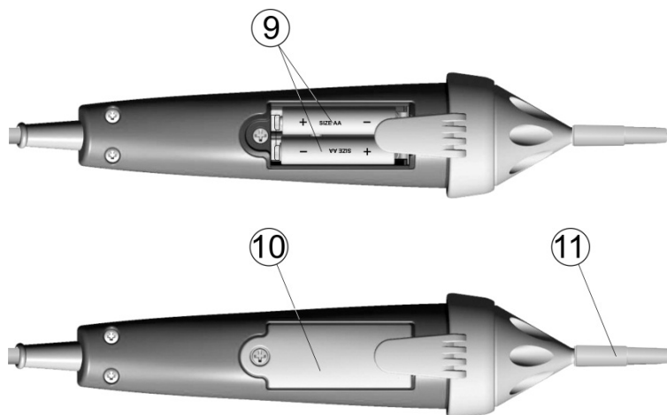
Abbildung C.3: Rückseite
