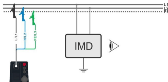
Abbildung 7.82: AUTO IT-Messung
