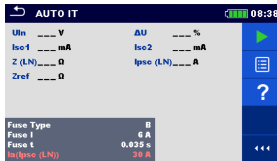
Abbildung 7.9: Menü AUTO IT
