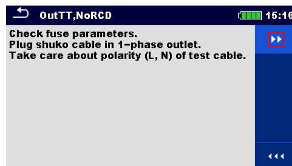
Abbildung 8.5: Auto Sequence® – Beispiel für Pause mit Hinweistext
