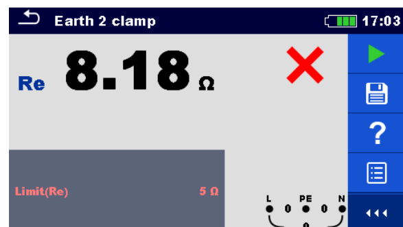
Abbildung 7.52: Beispiele für Ergebnisse der Erdungsmessung mit 2 Stromzangen
