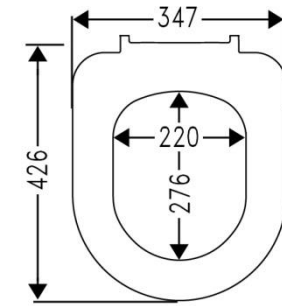
Gesamthöhe: 43mm
