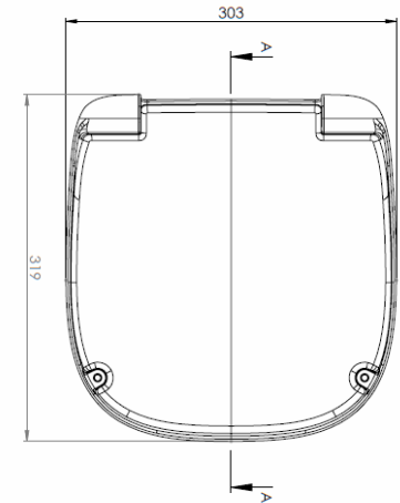
Gesamthöhe: 41mm
