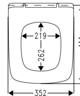
Gesamthöhe: 42 mm
