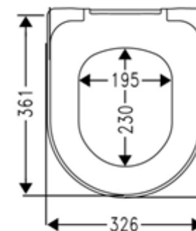
Gesamthöhe: 43mm
