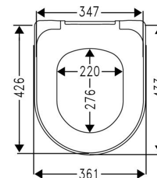
Gesamthöhe: 45mm
