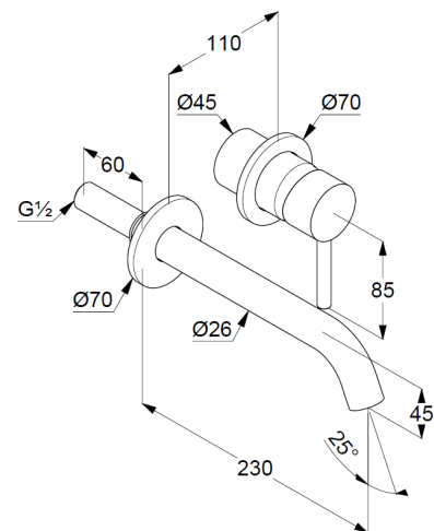
Maßzeichnung
