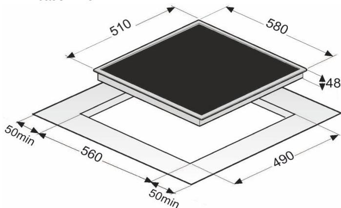
Einbauskizze
