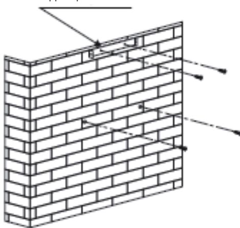
Support pour l'élément cheminée intérieur
