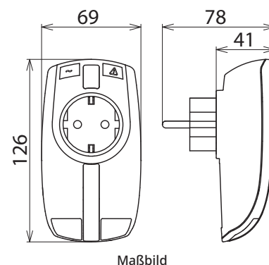
Maßbild
