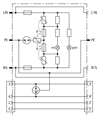
Prinzipschaltbild
