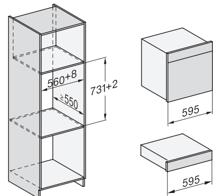
Einbau_DGC_XXL_ESW7x10_EVS7010, Skizze
