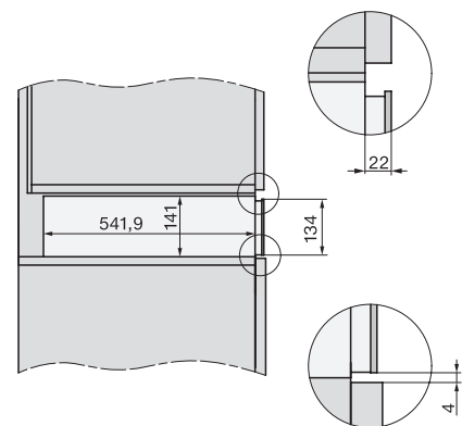
Seitenansicht ESW7x10 EVS7010, Skizze
