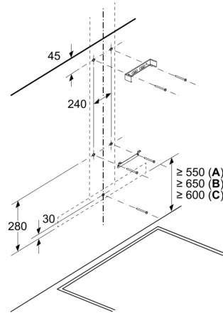
Maße in mm Wandinstallation mit Kamin
