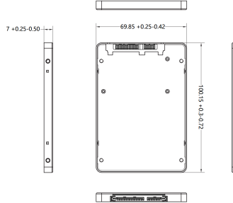
图1-1 结构尺寸（单位：mm）
