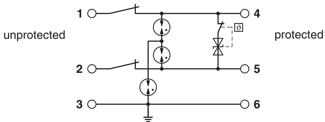
Schaltplan
