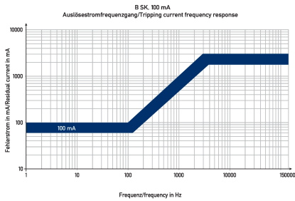
Kennlinie B SK 100 mA
