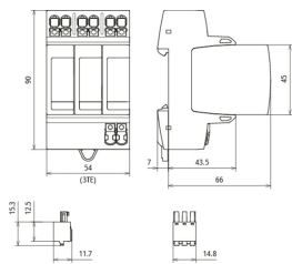
Maßbild DG MP YPV 1200 FM
