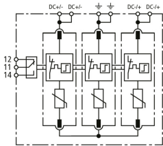
Prinzipialschaltbild DG MP YPV 1200 FM
