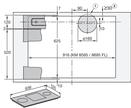
DAD4970, DAD6980, aufliegende Installation, gemeinsamer Ausschnitt, Skizze
