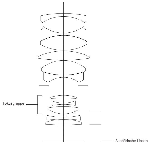
LINSENSCHNITT
