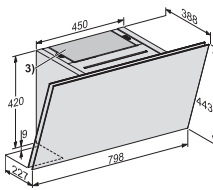
DAH2860 Skizze
