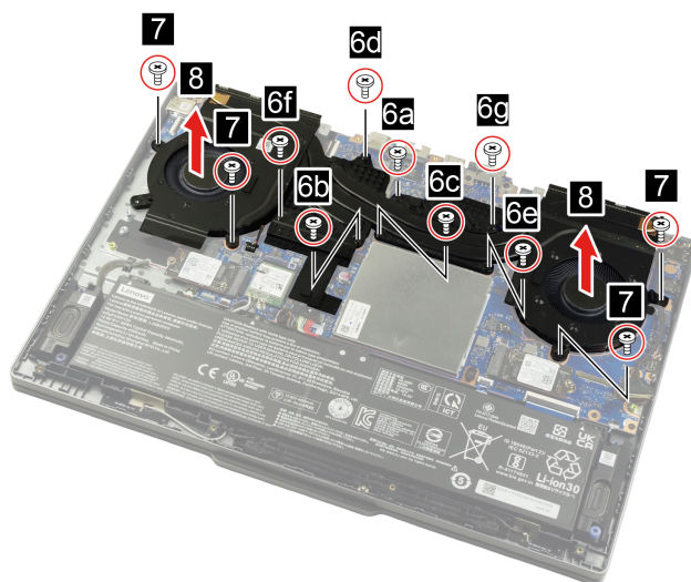
Figure 23. Remove the thermal module
