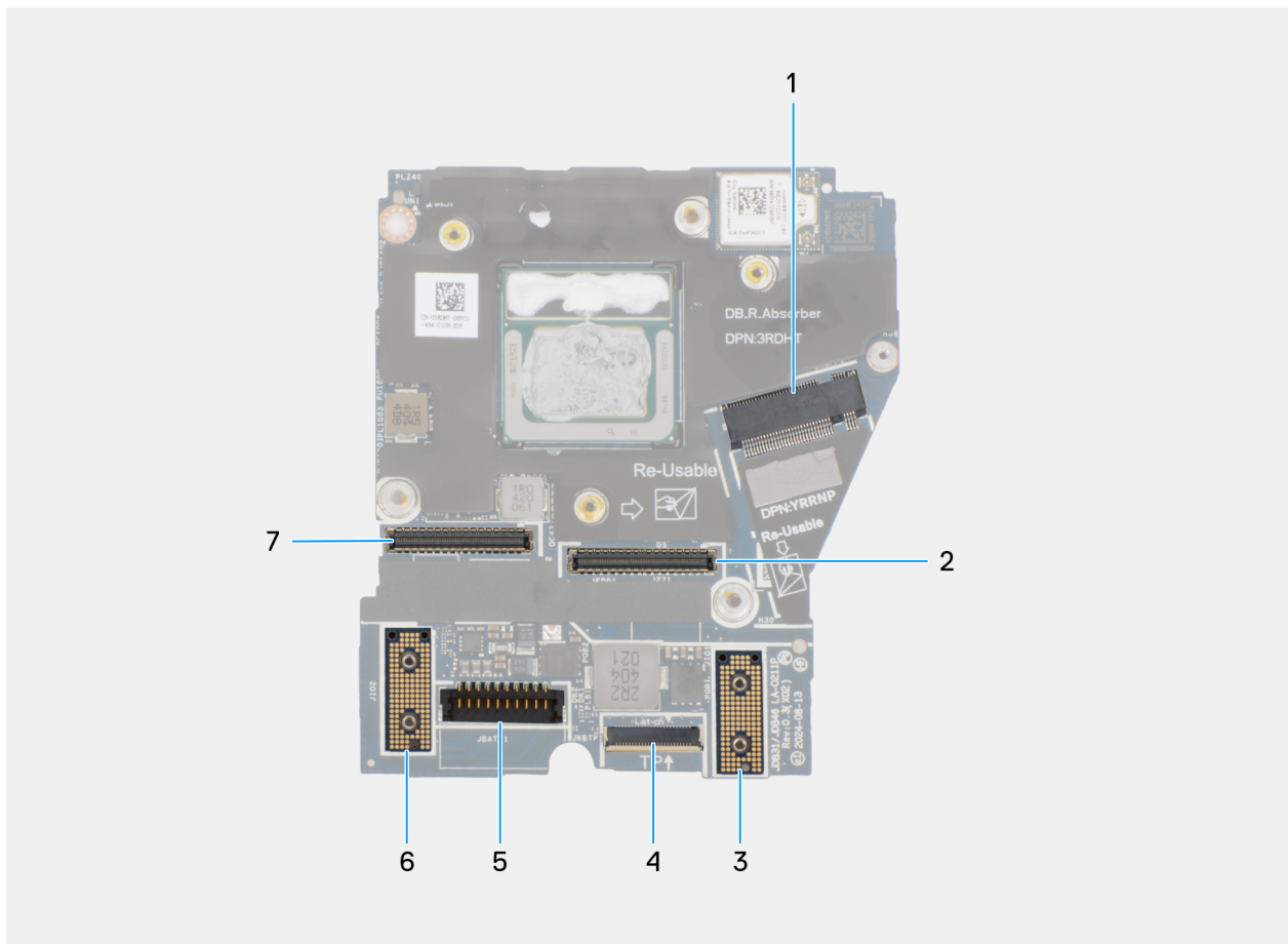
Abbildung 61. Komponenten auf der Hauptplatine
