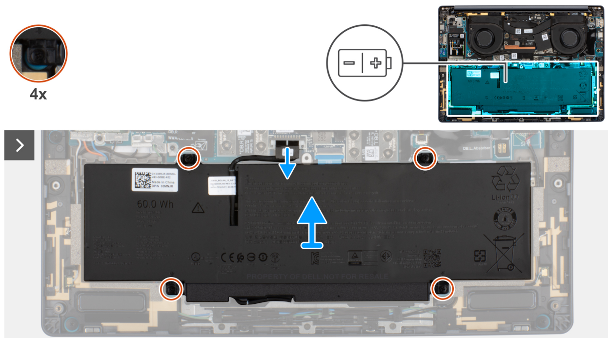
Abbildung 20. Lösen der unverlierbaren Schrauben
