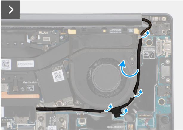
Abbildung 28. Entfernen des linken Lüfters
