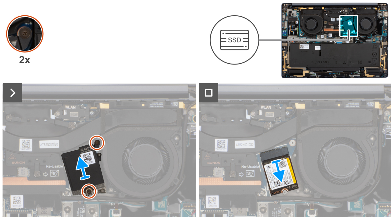
Abbildung 24. Entfernen des SSD
