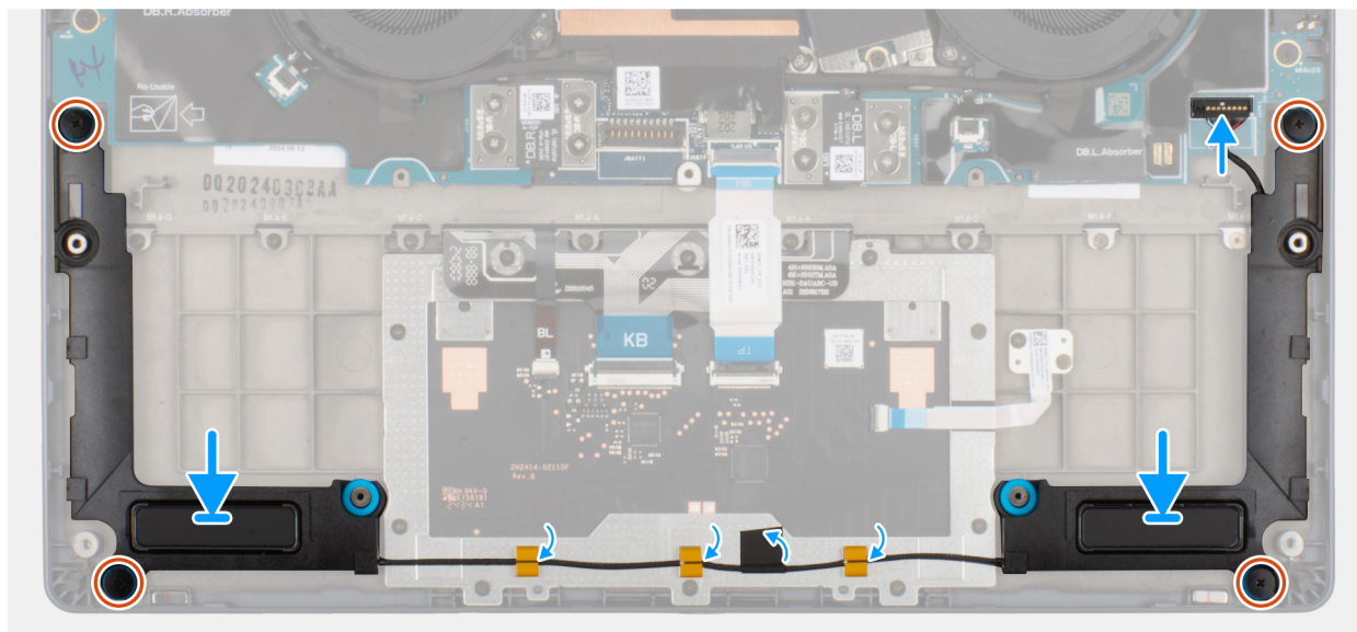
Abbildung 33. Einbauen der Lautsprecher ohne Antenne
