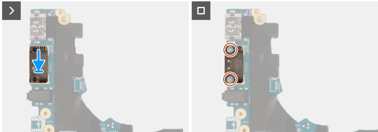
Abbildung 53. Installieren des rechten USB Typ-C-Moduls
