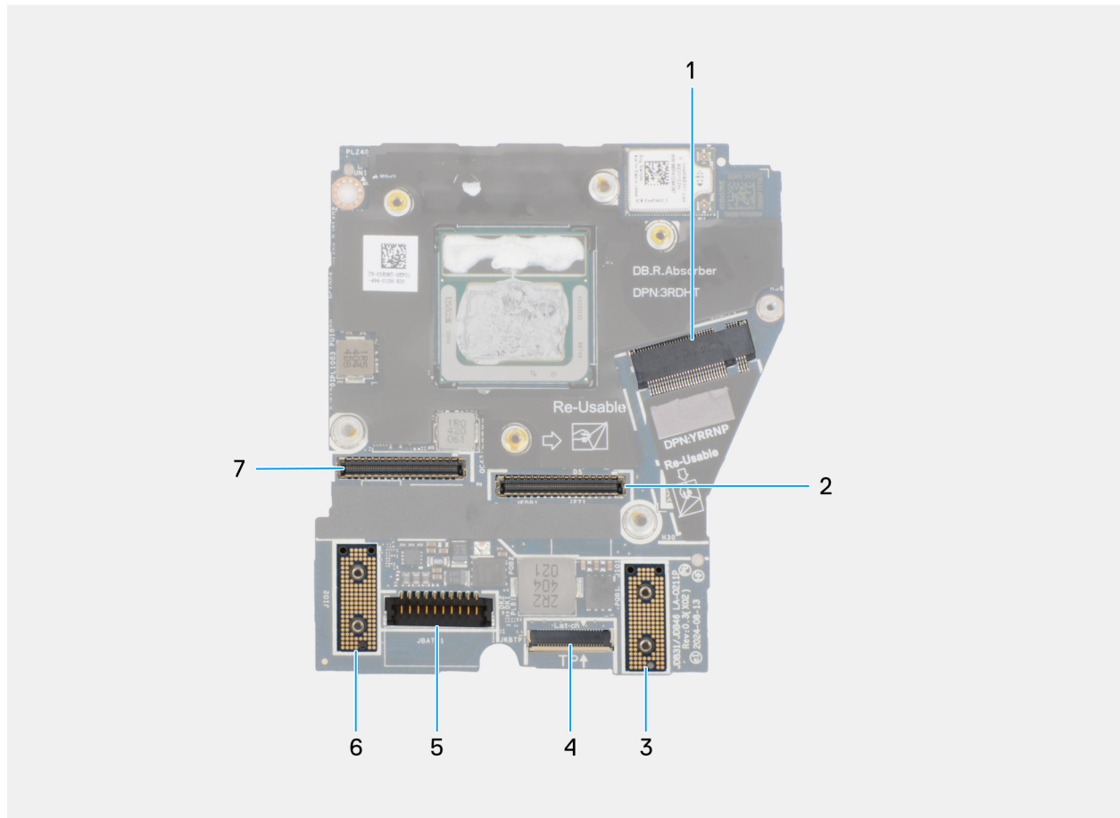
Abbildung 66. Komponenten auf der Hauptplatine
