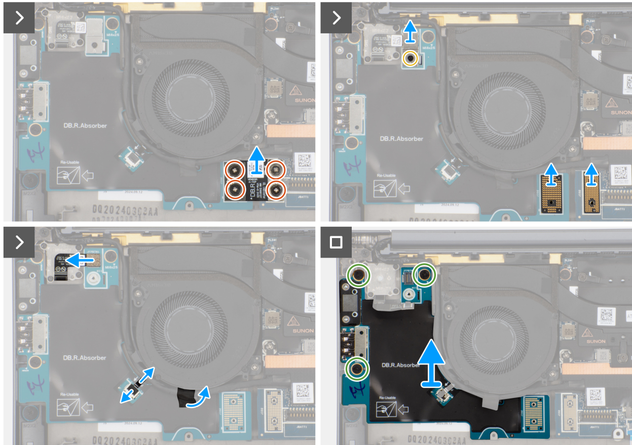
Abbildung 42. Entfernen der rechten I/O-Platine (ohne WWAN-Antennen)
