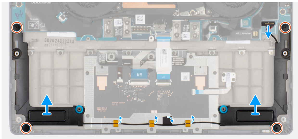
Abbildung 32. Entfernen der Lautsprecher ohne Antenne (WLAN-Konfiguration)
