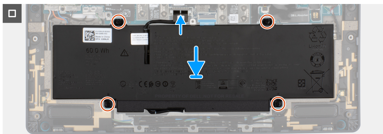
Abbildung 23. Einsetzen des Akkus
