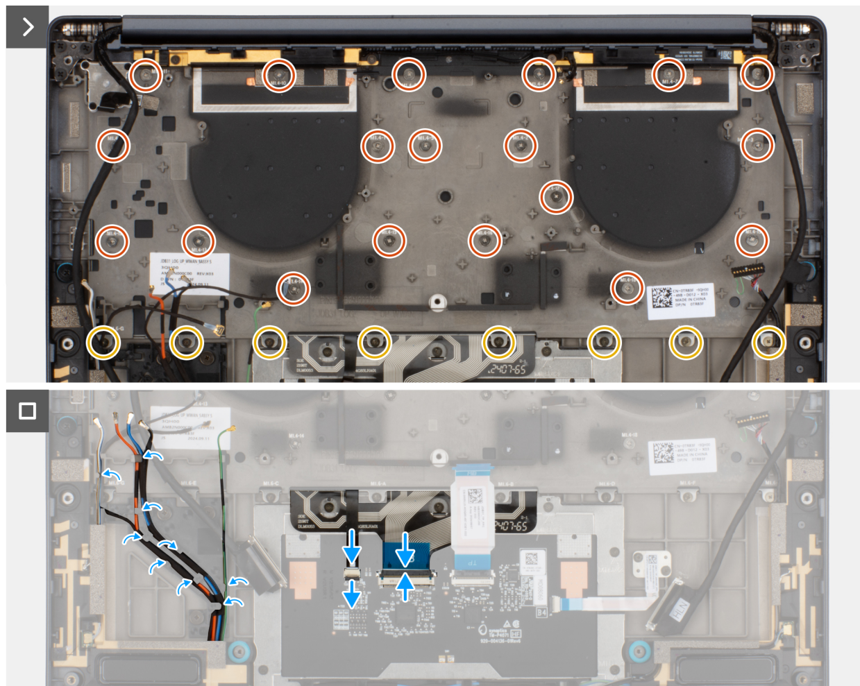
Abbildung 74. Installieren der Tastaturbaugruppe
