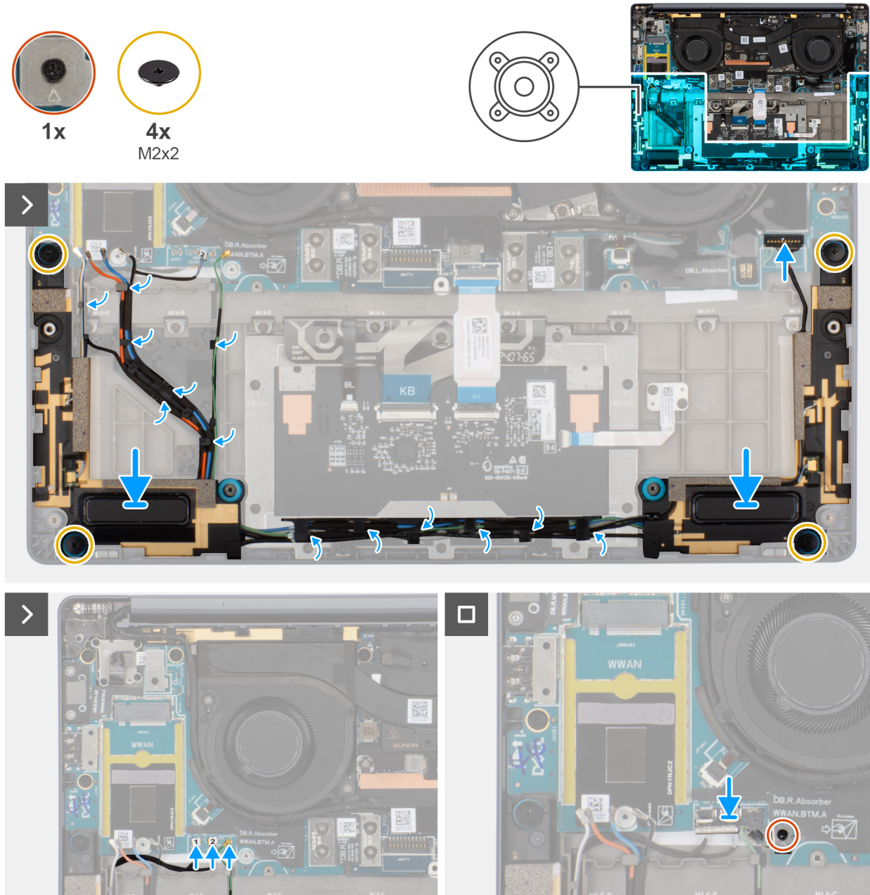
Abbildung 35. Installieren der Lautsprecher mit Antennen (WWAN-Konfiguration)
