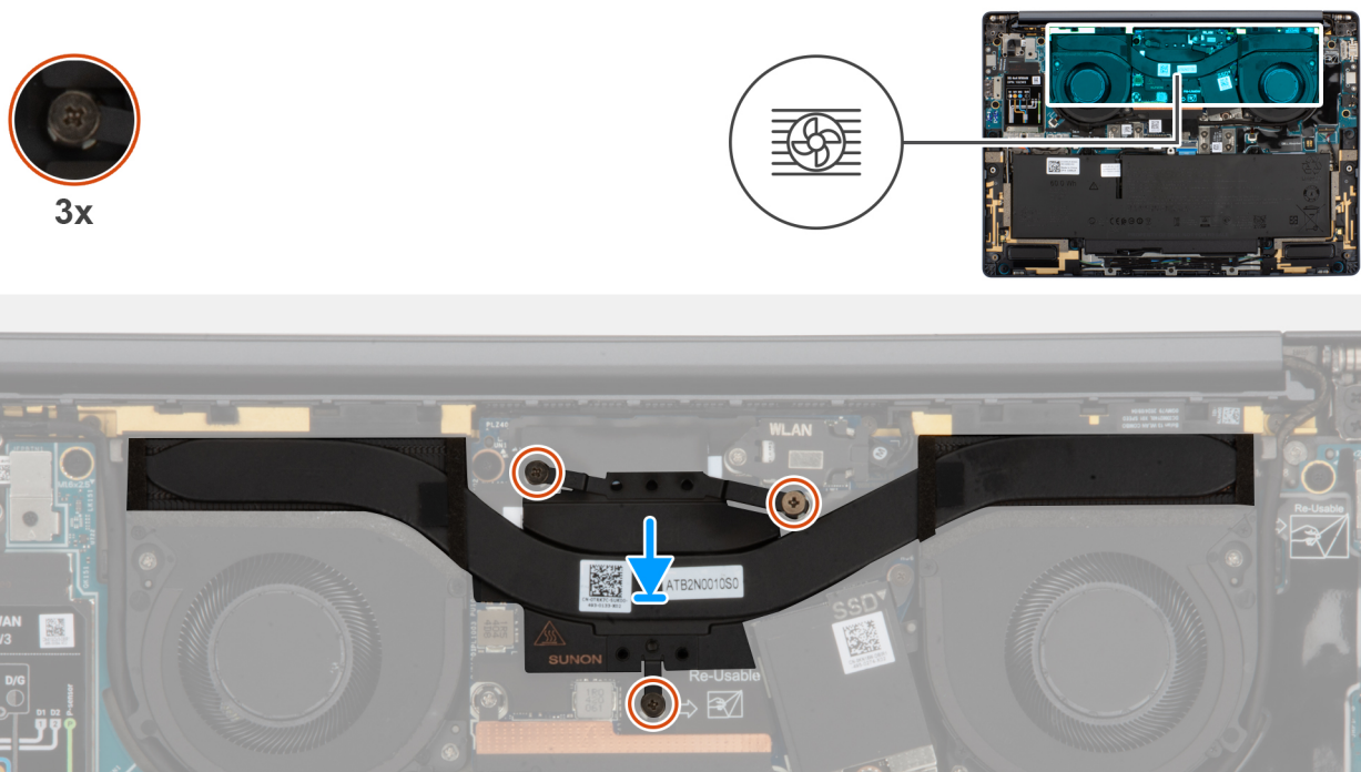
Abbildung 37. Einsetzen des Kühlkörpers
