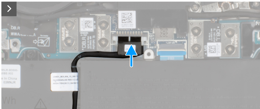
Abbildung 17. Verbinden des Batteriekabels mit der Hauptplatine
