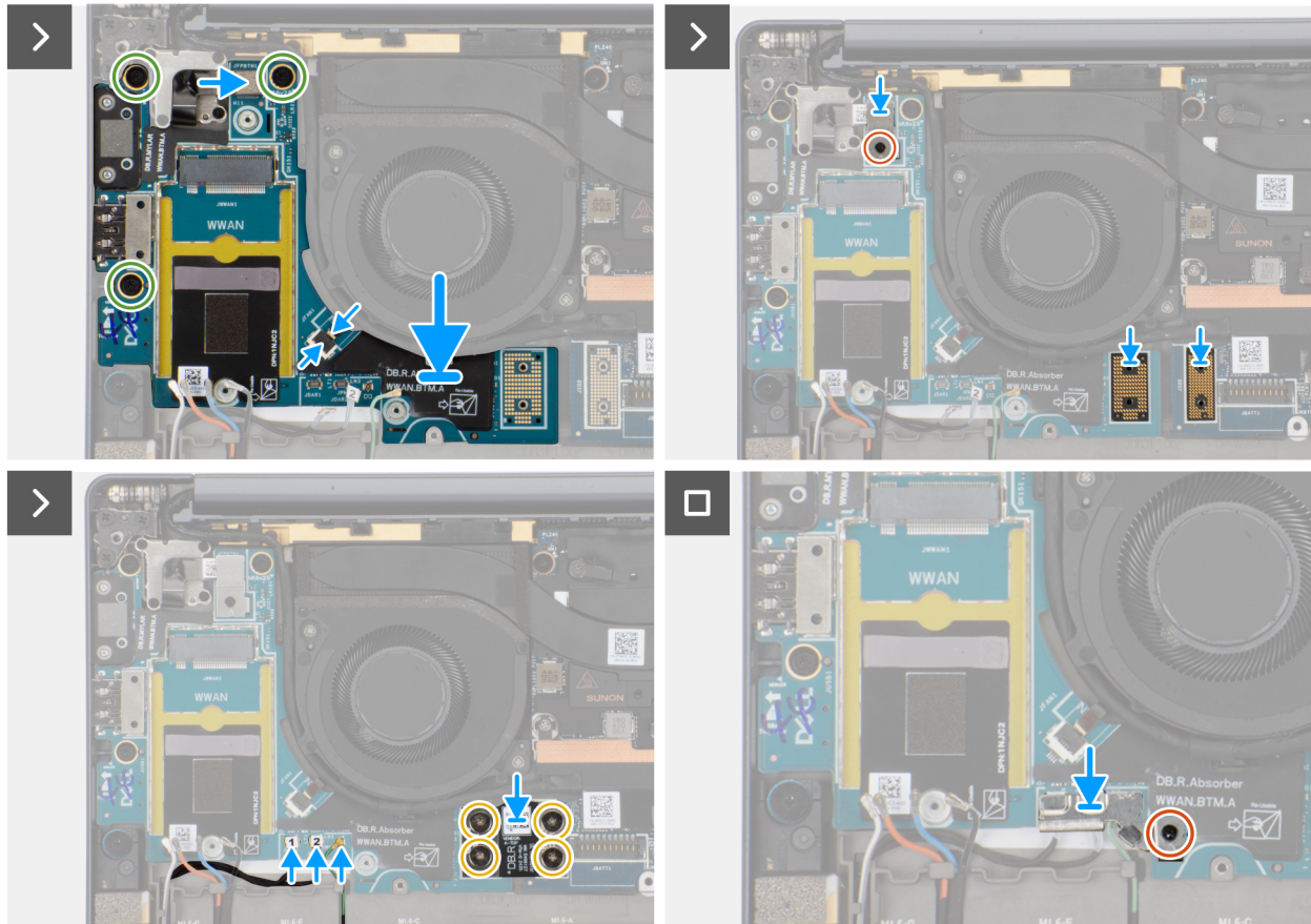
Abbildung 48. Installieren der rechten I/O-Platine (mit WWAN)
