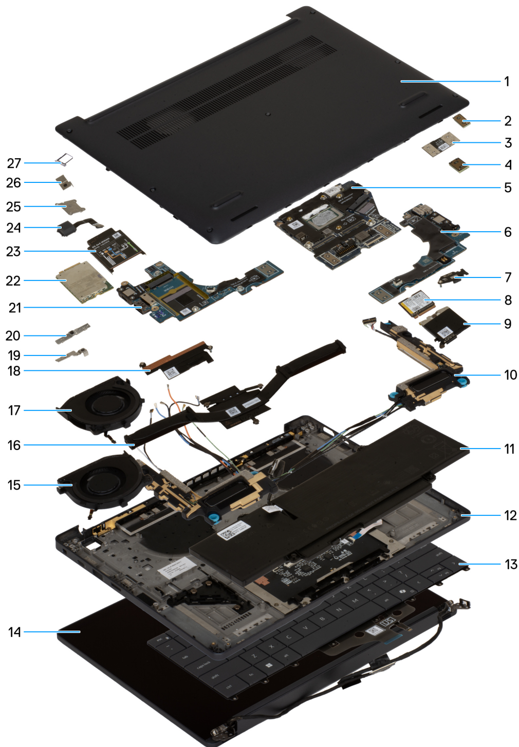
Abbildung 9. Hauptkomponenten Ihres Systems/Explosionsansicht
