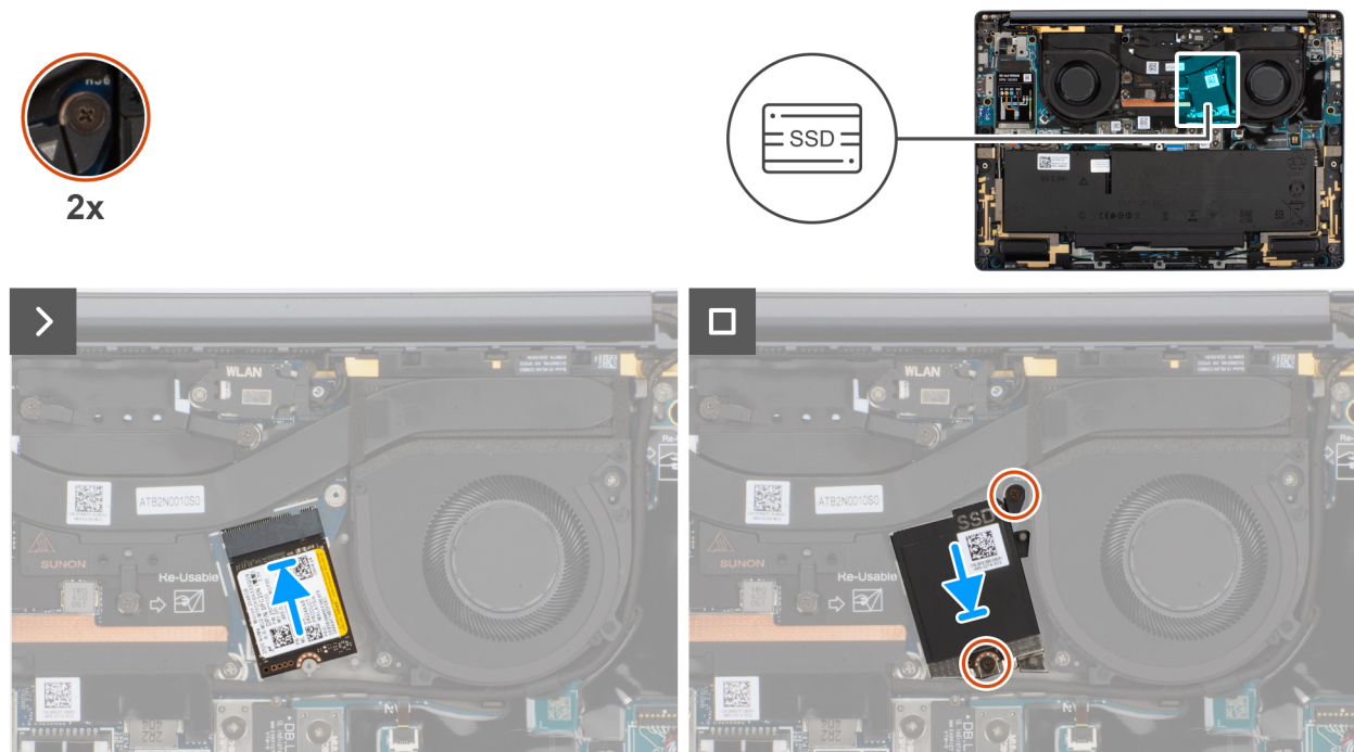
Abbildung 25. Einbauen der SSD-Karte
