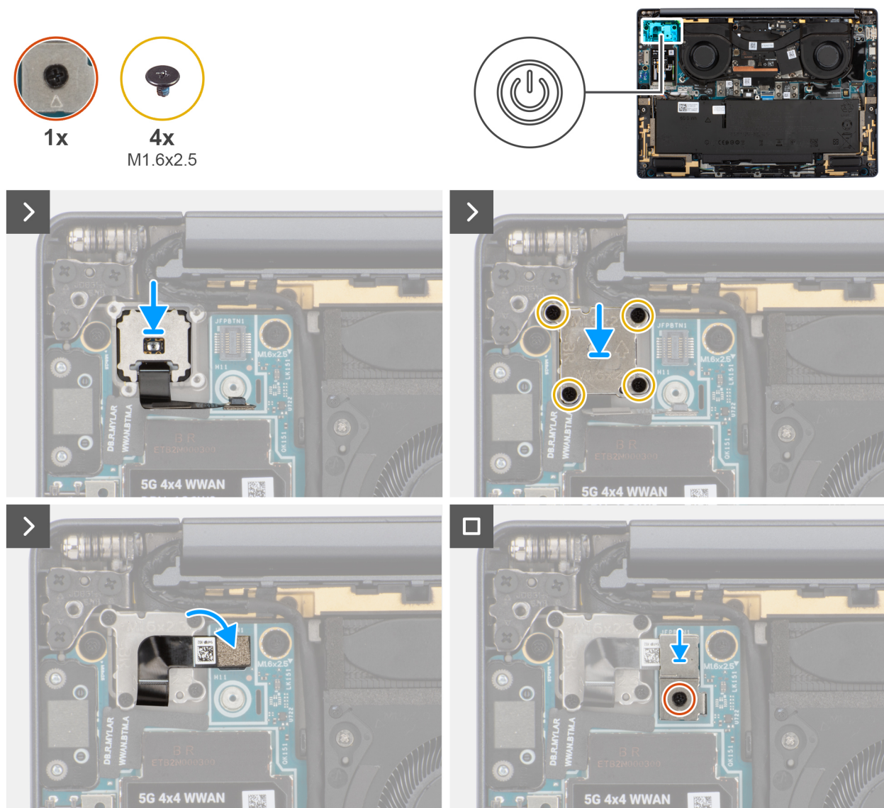
Abbildung 55. Installieren des Netzschalters
