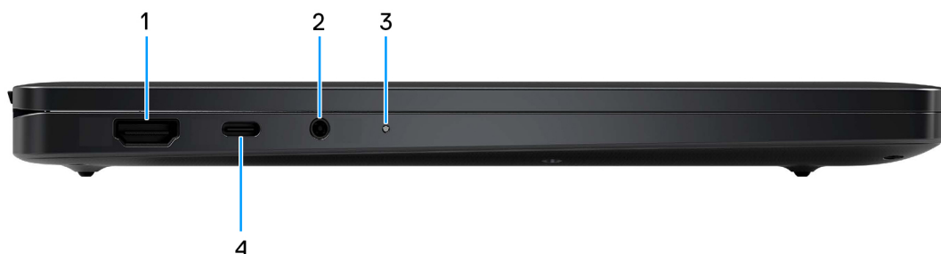
Abbildung 2. Linke Seitenansicht
