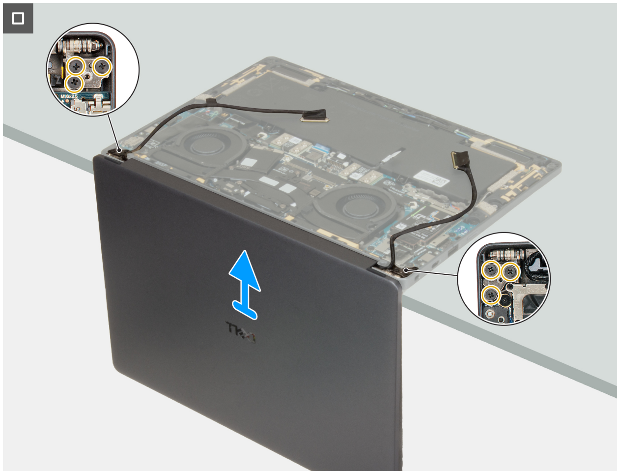
Abbildung 57. Entfernen der Bildschirmbaugruppe
