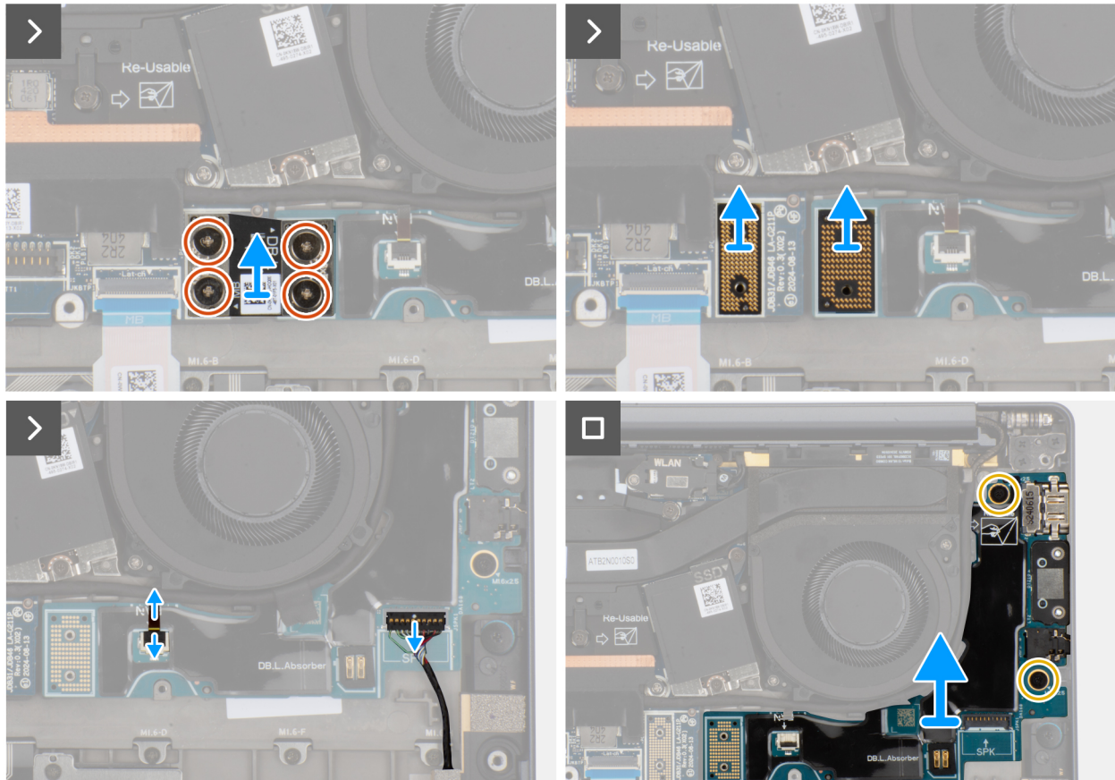
Abbildung 38. Entfernen der linken E/A-Platine
