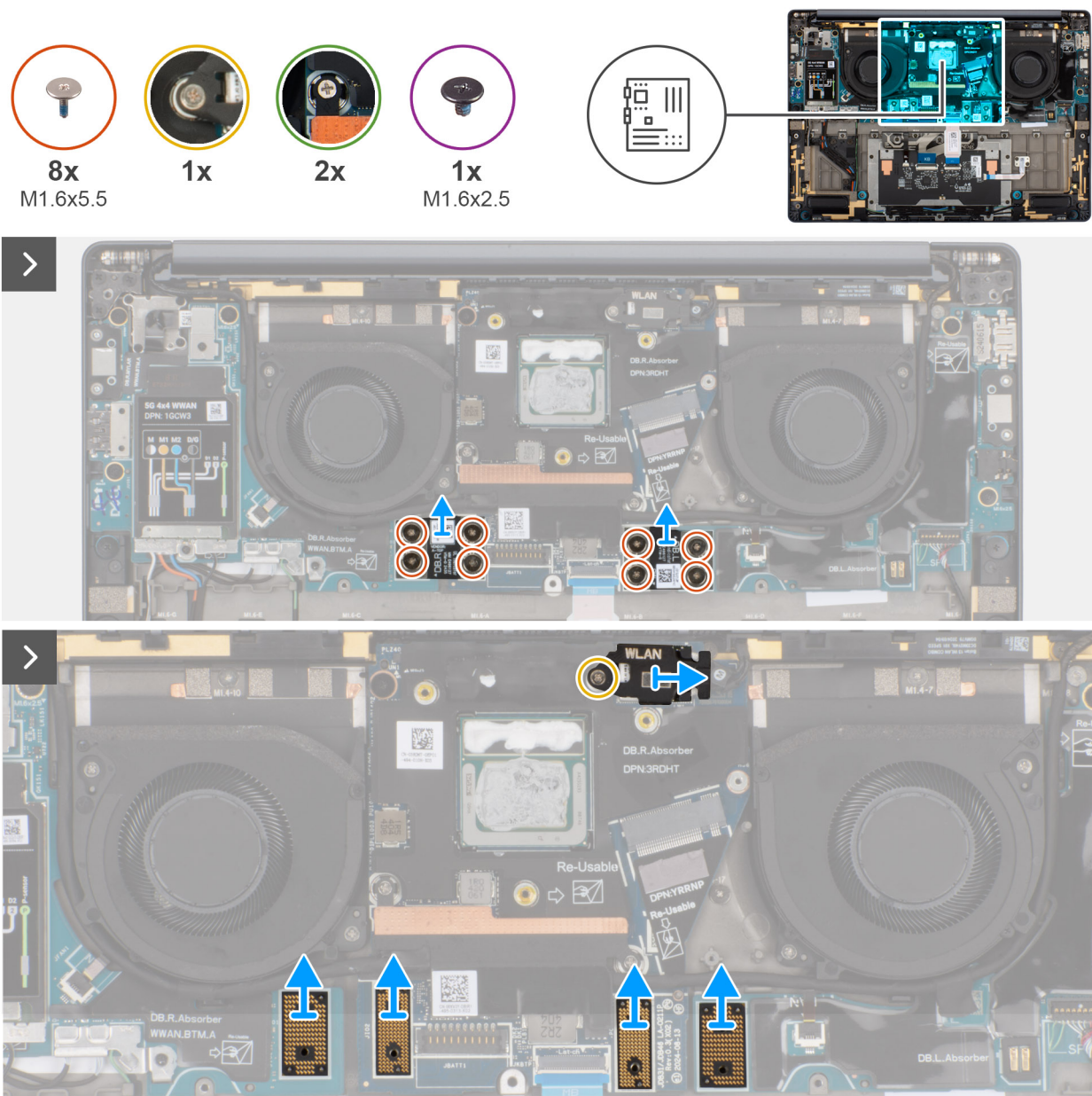
Abbildung 62. Entfernen der Systemplatine
