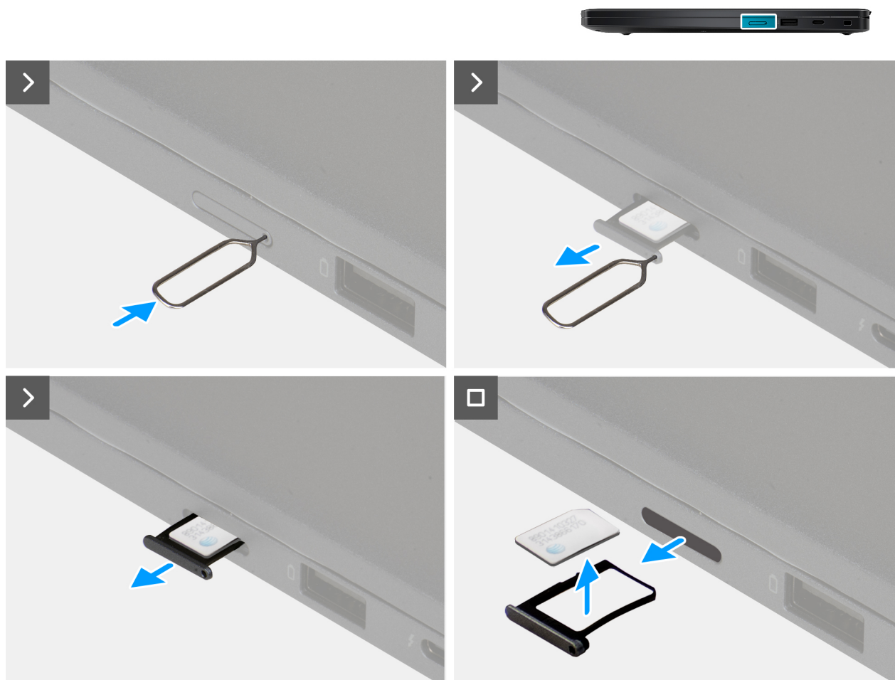
Abbildung 12. Entfernen der Nano-SIM-Karte
