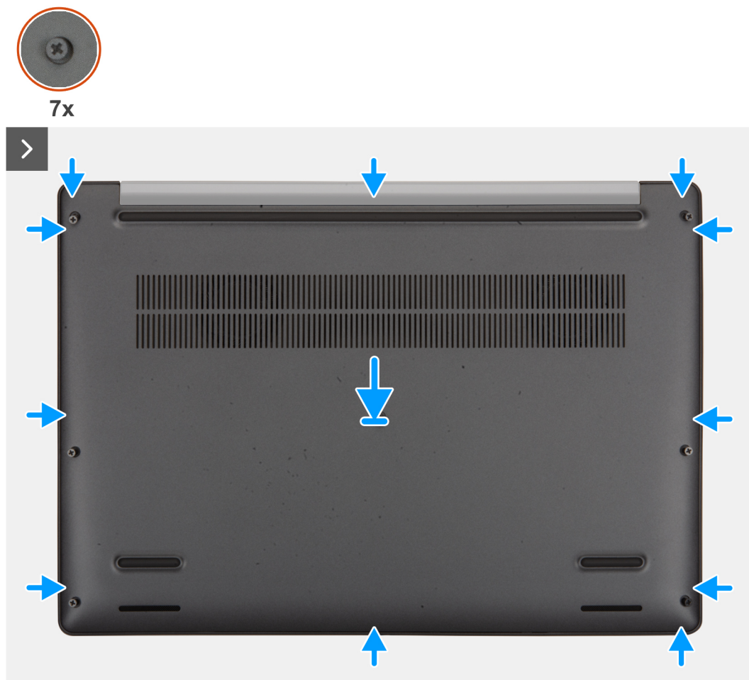
Abbildung 18. der Bodenabdeckung
