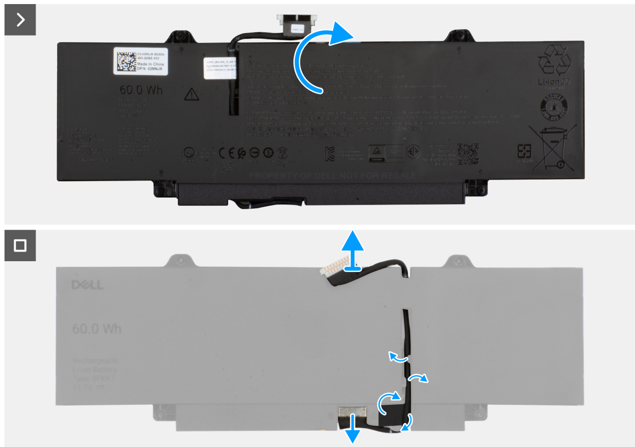
Abbildung 21. Entfernen des Akkus und Trennen des Batteriekabels
