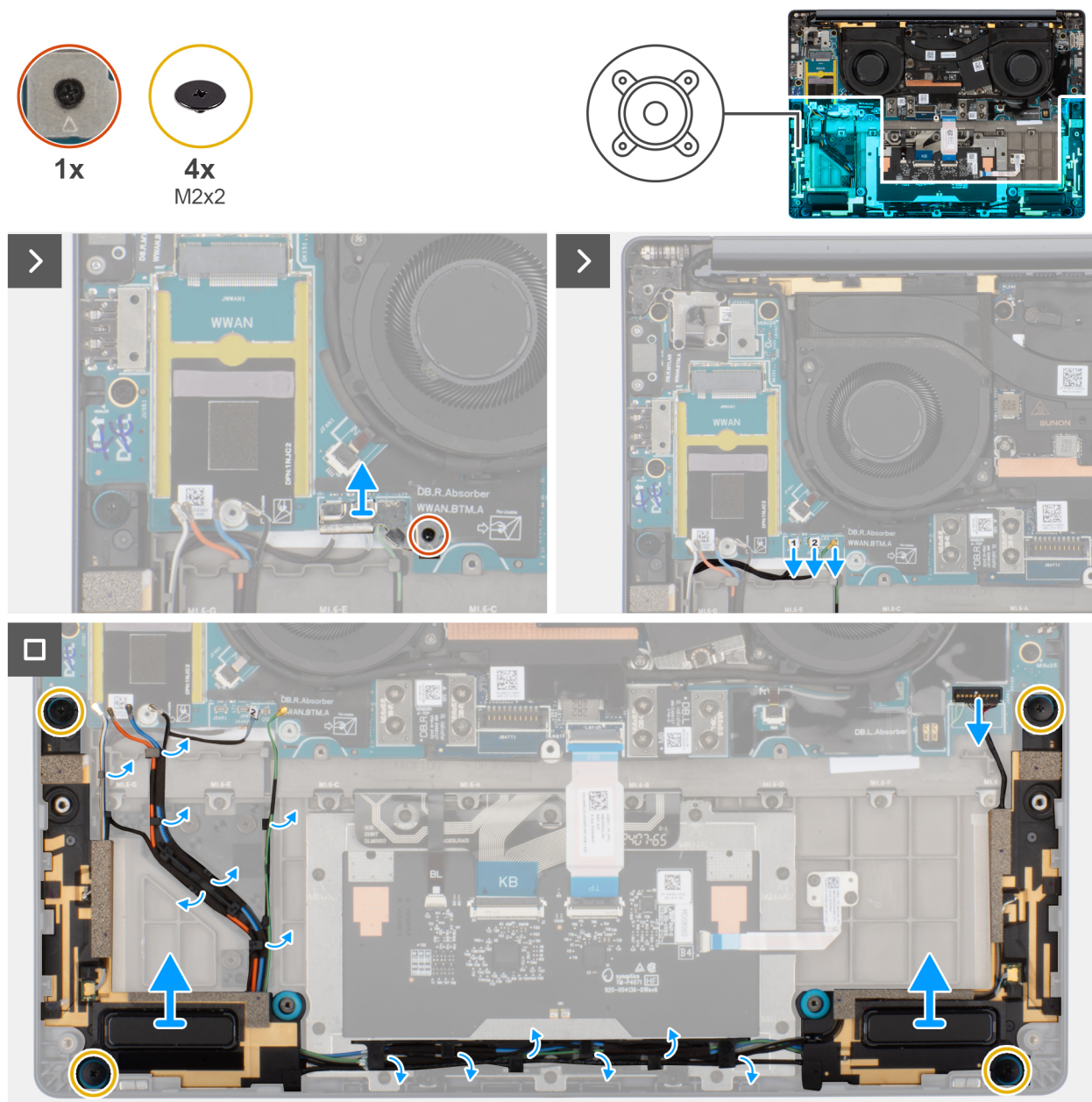
Abbildung 34. Entfernen der Lautsprecher mit Antennen (WWAN-Konfiguration)
