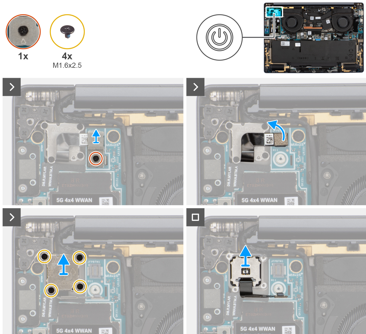
Abbildung 54. Entfernen des Netzschalters
