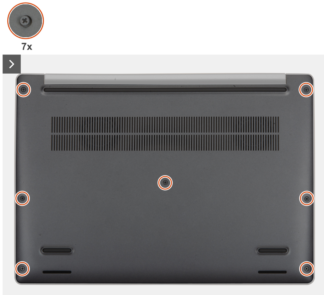
Abbildung 14. Lösen der unverlierbaren Schrauben
