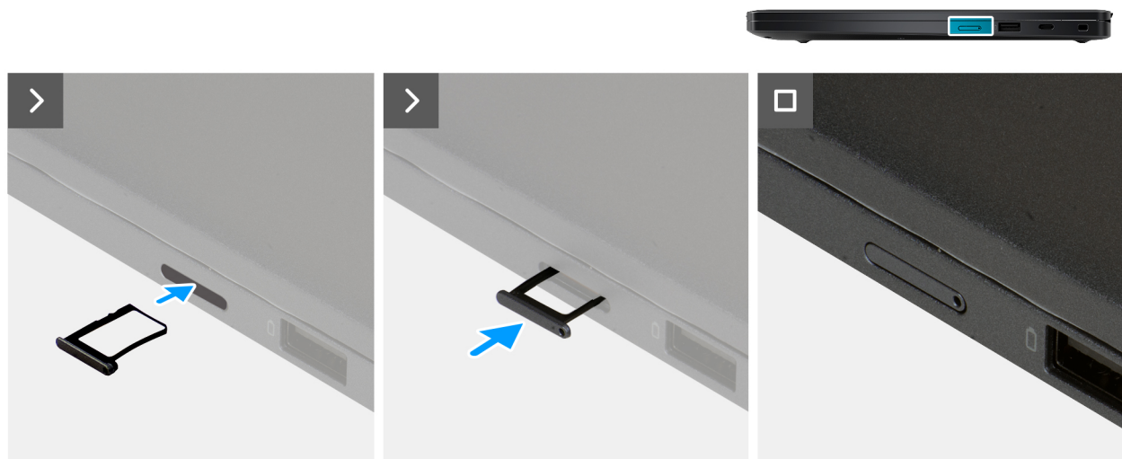
Abbildung 11. Installieren des Nano-SIM-Kartenfachs
