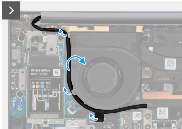
Abbildung 30. Entfernen des rechten Lüfters
