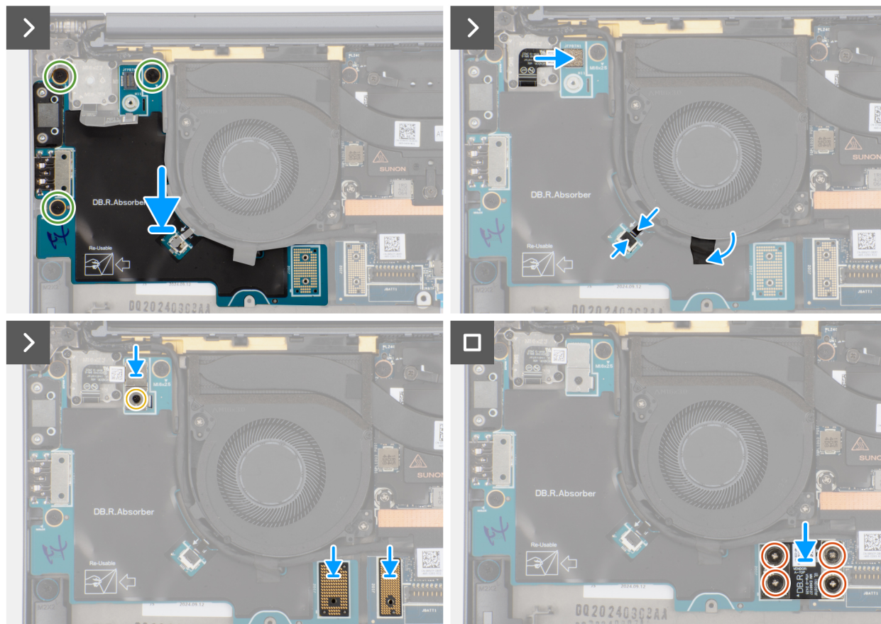
Abbildung 44. Installieren der rechten I/O-Platine (ohne WWAN-Antennen)
