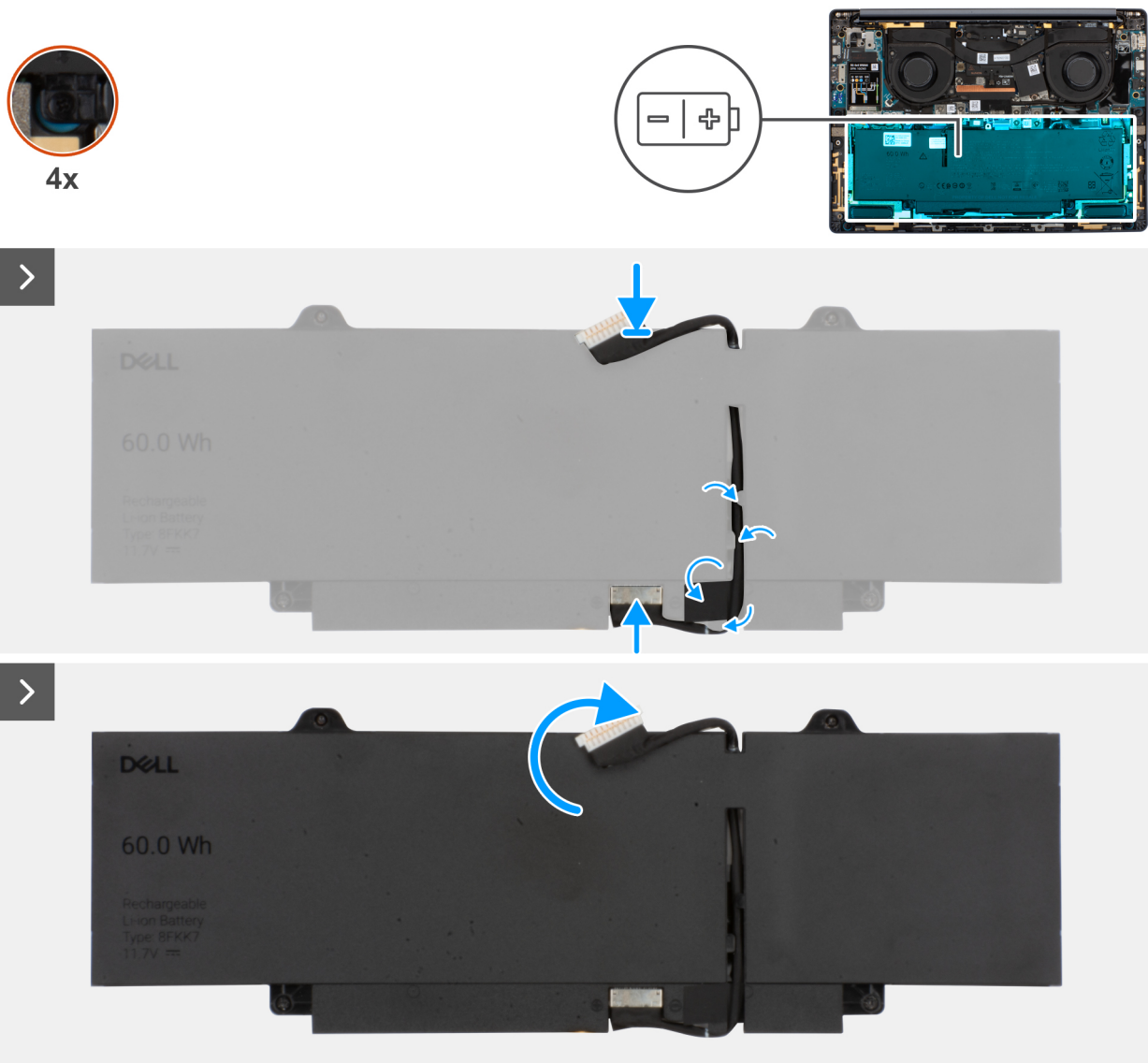
Abbildung 22. Verbinden des Akkukabels
