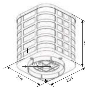
Maßzeichnung Plasmafilter PLS620
