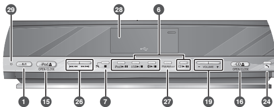
Face avant
