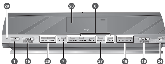
Frontvy
