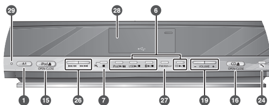
Vooraangezicht
