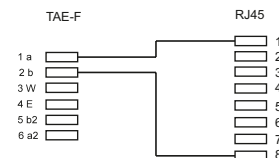
Goobay TAE Adapter TAE-F-Stecker > RJ45-Buchse (8P2C) • TAE PIN 1(a) -> RJ 45 PIN 1, TAE PIN 2(b) -> RJ 45 PIN 8 • passend für FRITZ Box
