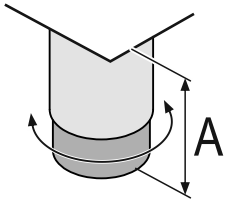
Fig. 10 Der Stellfuß ist von A = 115 mm (4 1/2 in) bis 175 mm (6 7/8 in) verstellbar.
