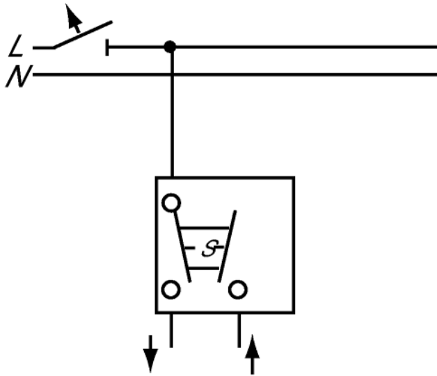
Anschlussbild
