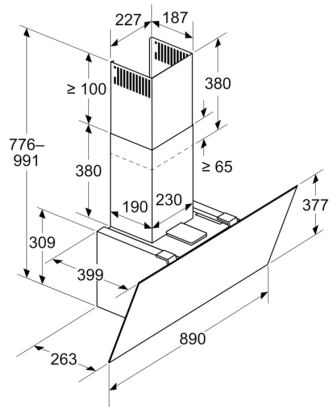
Maße in mm Gerät im Umluftbetrieb
