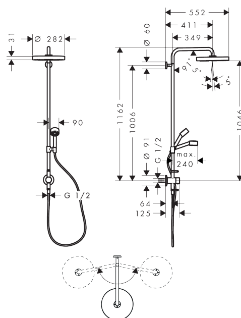
Maßzeichnung
