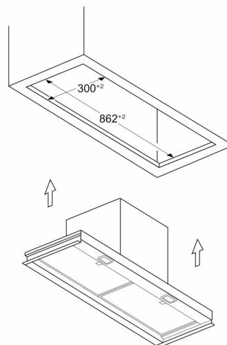
Maße in mm Einbaubeispiel in Möbelausschnitt
