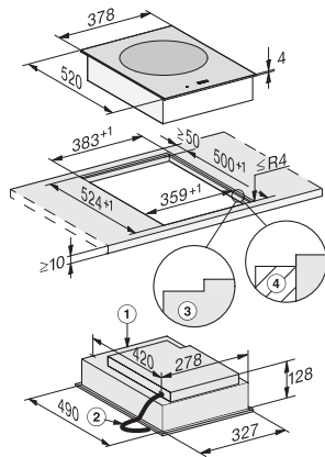
CS7641FL, flächenbündig (*Fußnote) (Skizze)
