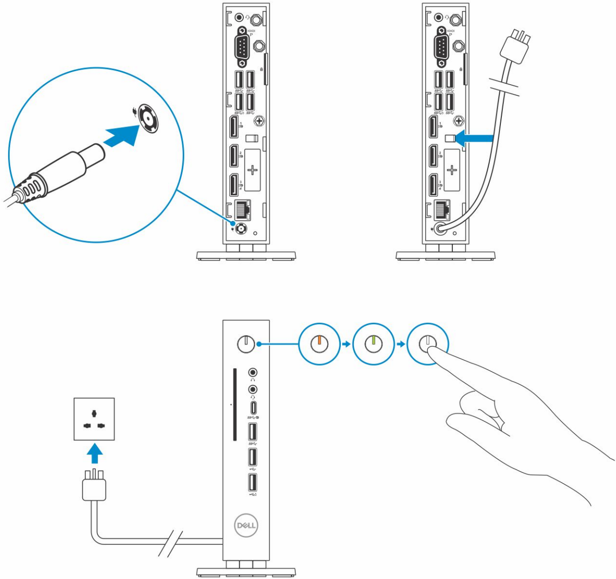
Abbildung 6. Stromkabel anschließen
