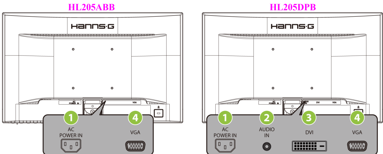
ABBILDUNG 2. ANSCHLISSEN AN EINEN PC
