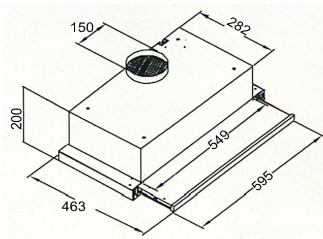
Einbauskizze
