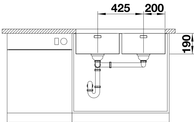
Frontansicht
