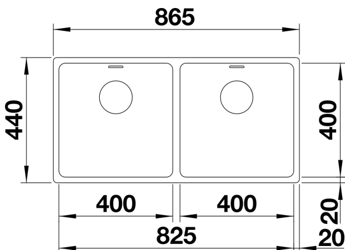
Aufsicht
