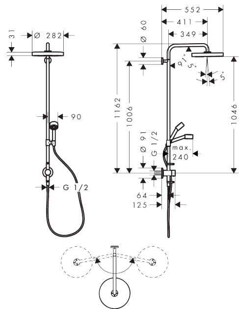
Maßzeichnung
