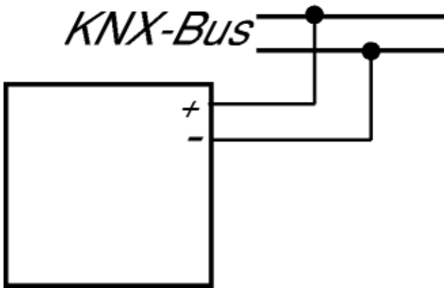
Anschlussbild
