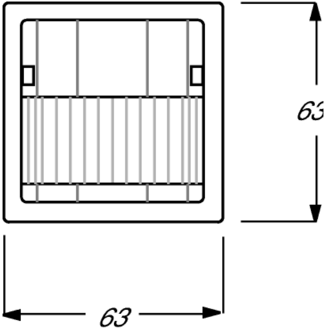
Maßbild
