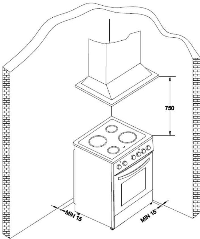
Abmessungen Gerät, in mm
