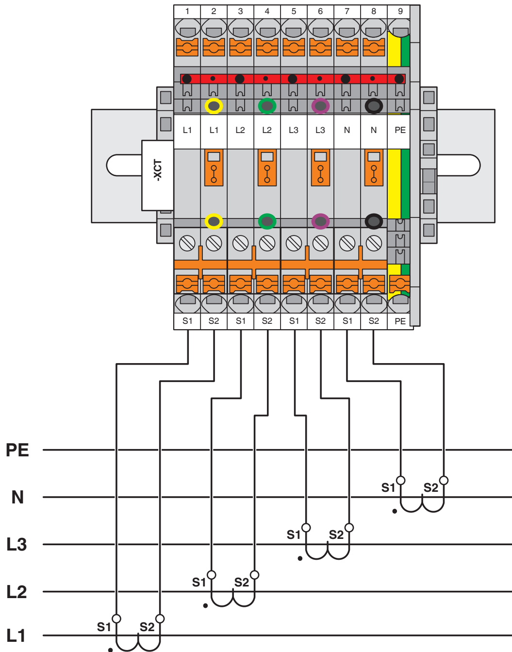
Schaltplan
