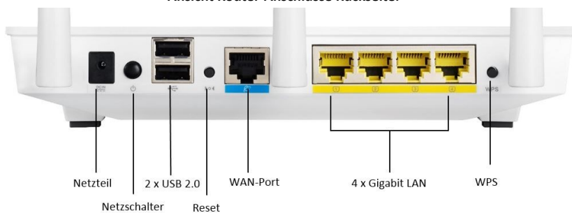
Ansicht Router-Anschlüsse Rückseite:
