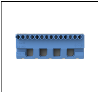
ZK144B N-Klemmenblock 14x4+4x25qmm EAN Art.-Nr. 2CPX062754R9999 Listenpreis 15.35 €
