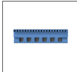
ZK206B N-Klemmenblock 20x4+6x25qmm EAN Art.-Nr. 2CPX062756R9999 Listenpreis 20.00 €
