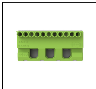
ZK113G PE-Klemmenblock 11x4+3x25qmm EAN Art.-Nr. 2CPX062759R9999 Listenpreis 11.95 €
