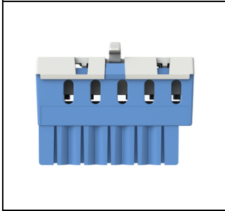
ZK50B N-Klemmenblock 5x4qmm EAN Art.-Nr. 2CPX062750R9999 Listenpreis 5.40 €
