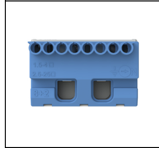
ZK82B N-Klemmenblock 8x4+2x25qmm EAN Art.-Nr. 2CPX062752R9999 Listenpreis 8.55 €
