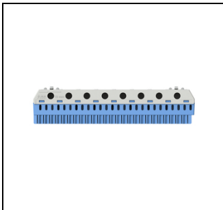
ZK268B N-Klemmenblock 23x4+7x25qmm EAN Art.-Nr. 2CPX063164R9999 Listenpreis 23,90 €
