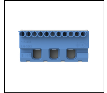
ZK113B N-Klemmenblock 11x4+3x25qmm EAN Art.-Nr. 2CPX062753R9999 Listenpreis 11.95 €
