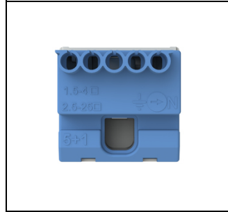
ZK51B N-Klemmenblock 5x4+1x25qmm EAN Art.-Nr. 2CPX062751R9999 Listenpreis 6.70 €
