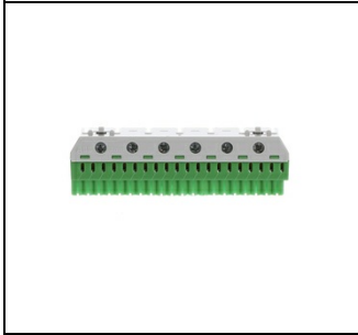
ZK206G PE-Klemmenblock 20x4+6x25qmm EAN Art.-Nr. 2CPX062762R9999 Listenpreis 20,00 €
